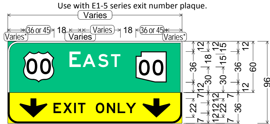
Var ; 32 ; 37.42 ; 12 ; 47.32 ; 32 ; Var E6-101ex (freeway - 36" shield)
