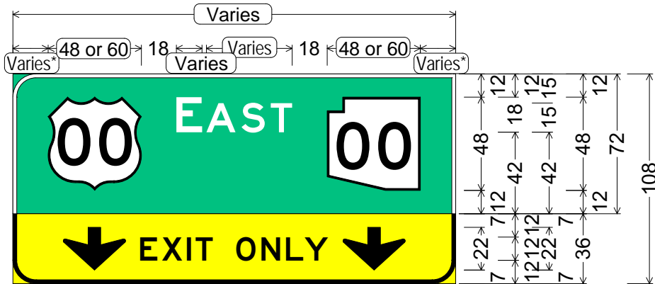
Var ; 32 ; 37.42 ; 12 ; 47.32 ; 32 ; Var E6-101ex (freeway - 48" shield option)
