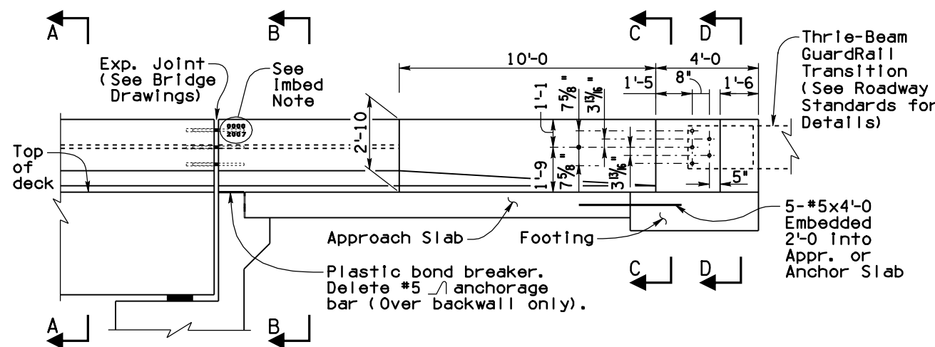
ELEVATION
