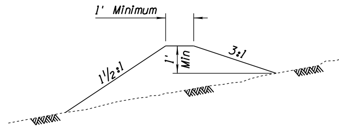
CROWN DIKE
