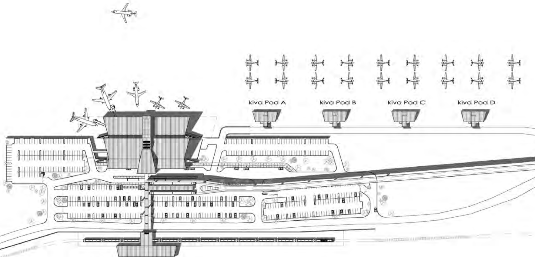
KIVA POD SITE PLAN
