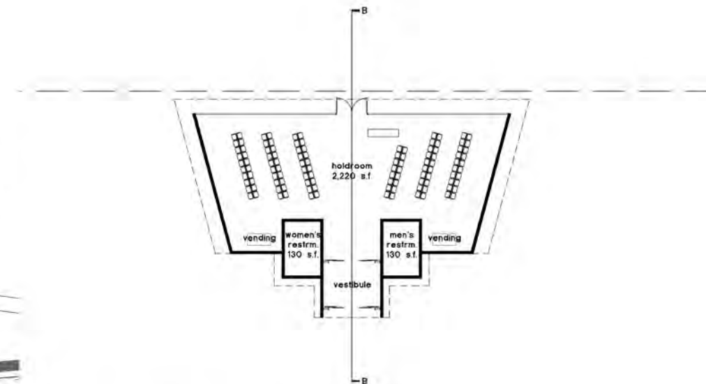
KIVA POD PLAN
