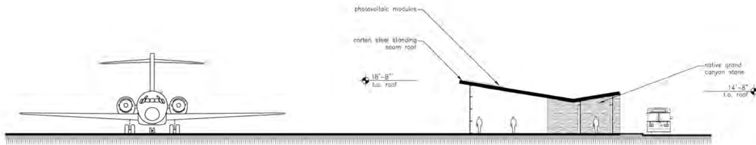
KIVA POD SECTION B-B
